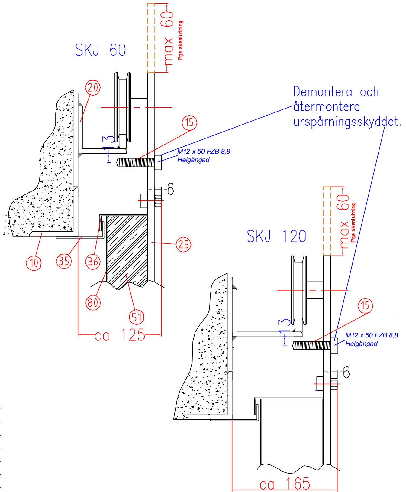
Bilaga 6 till monteringsinstruktion för brandskjutport A60 (E160) och E120 (A60/E160)
