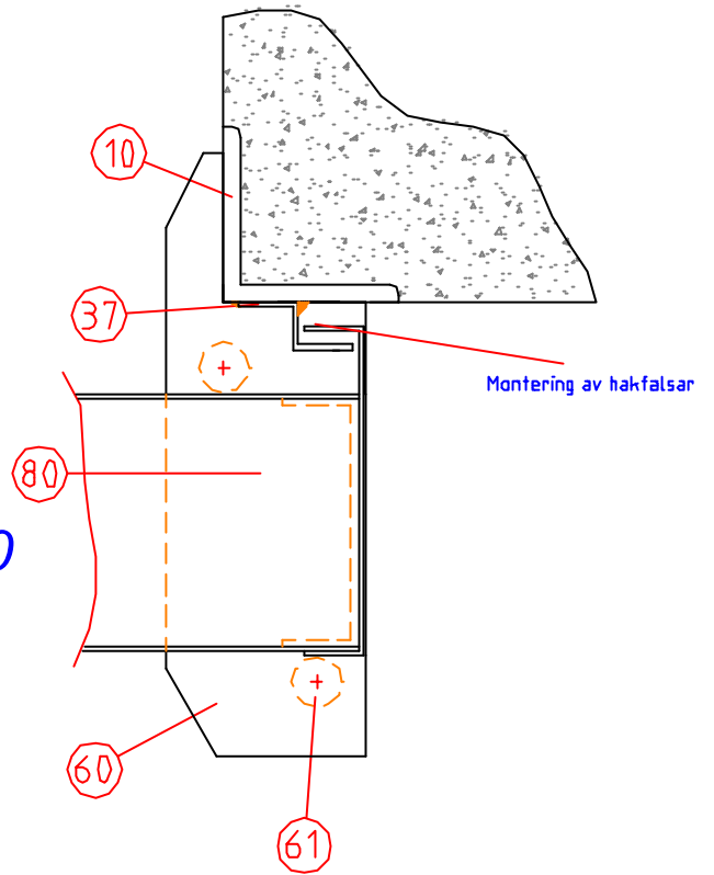
Bilaga 9 till montageinstruktion för brandskjutport A60 ( E160 ) och E120 ( A120/E1120 )
