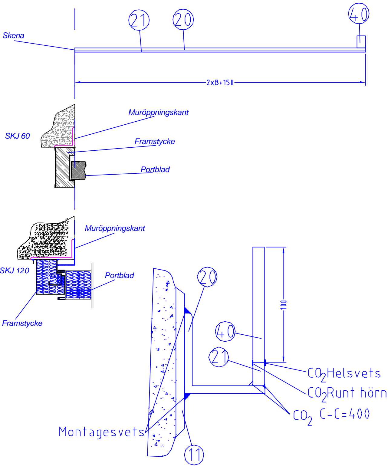
Bilaga 4 till montageinstruktion för brandskjutport A60 ( EI60 ) och E120 ( A120/EI120 )
